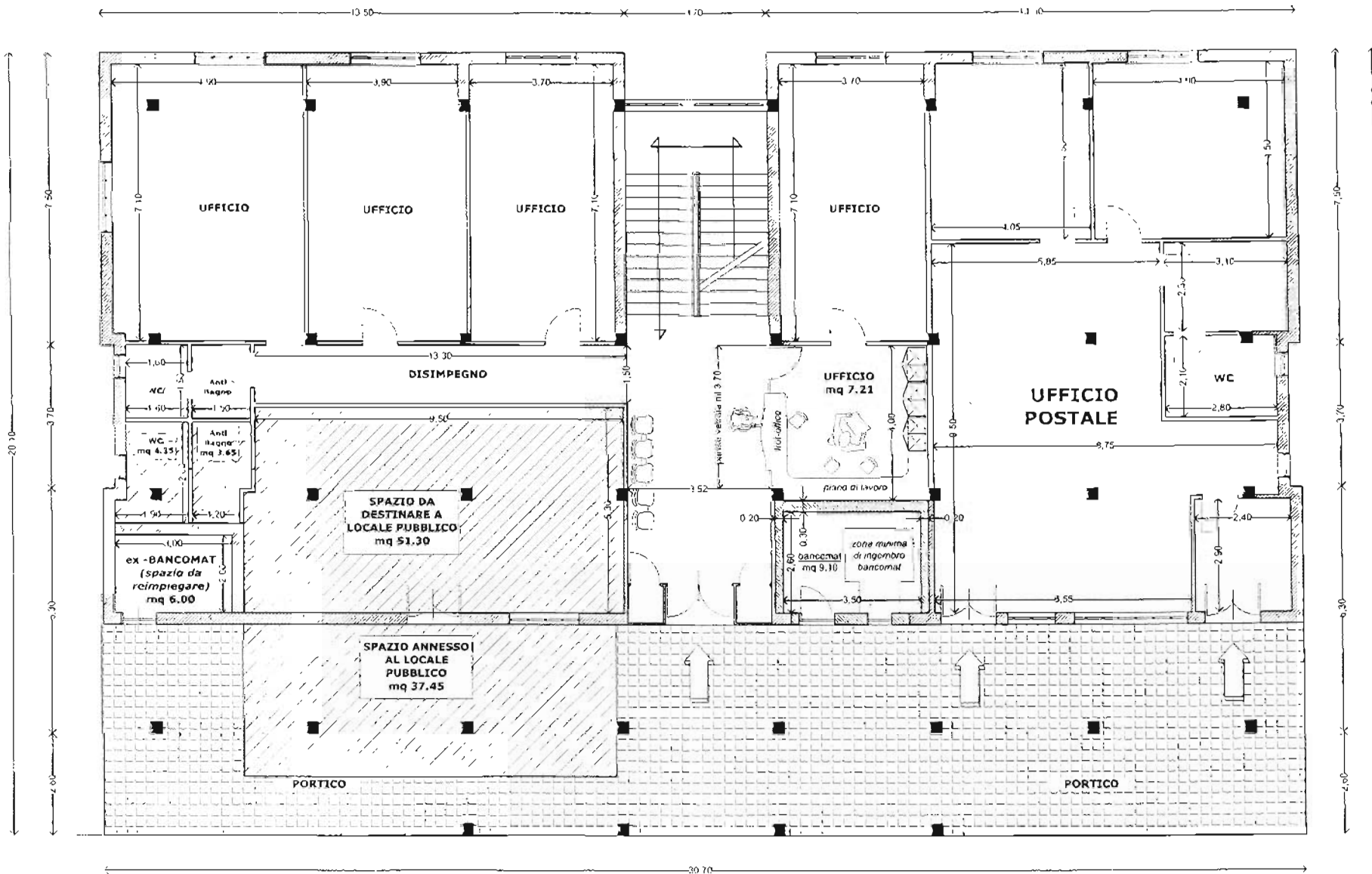
Planimetria di variazione PIANO TERRA (a quota Piazza Aldo Moro)
